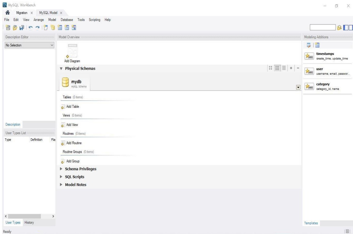
Fig: 3.4.6 Database
