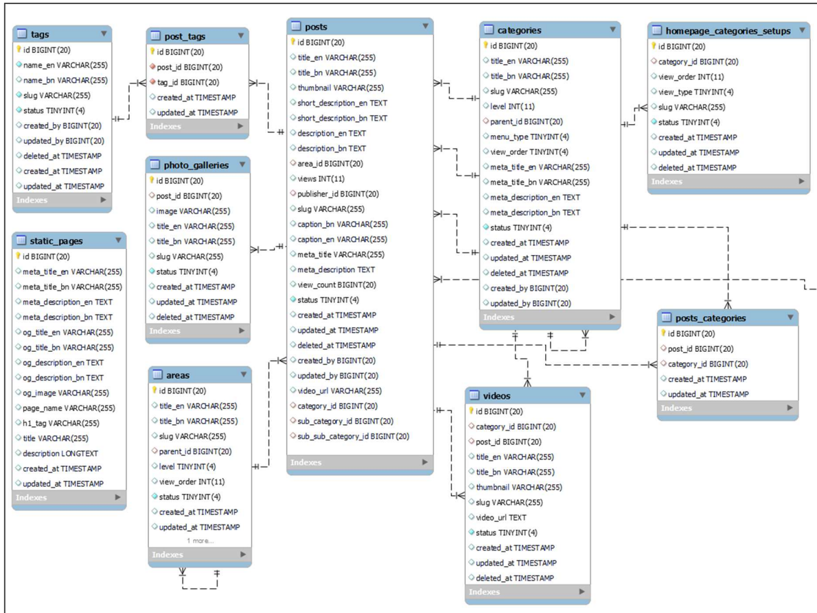
Fig 3.3 System ER diagram
