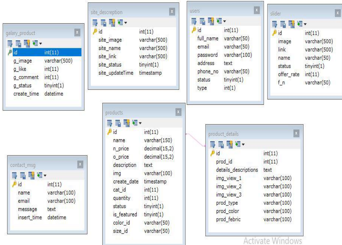
Fig: 3.17 Database Schema Design
