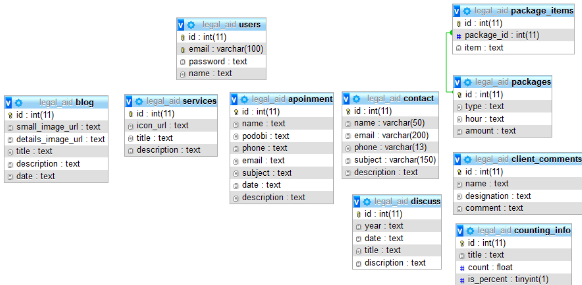
Figure 5.1: ER diagram
