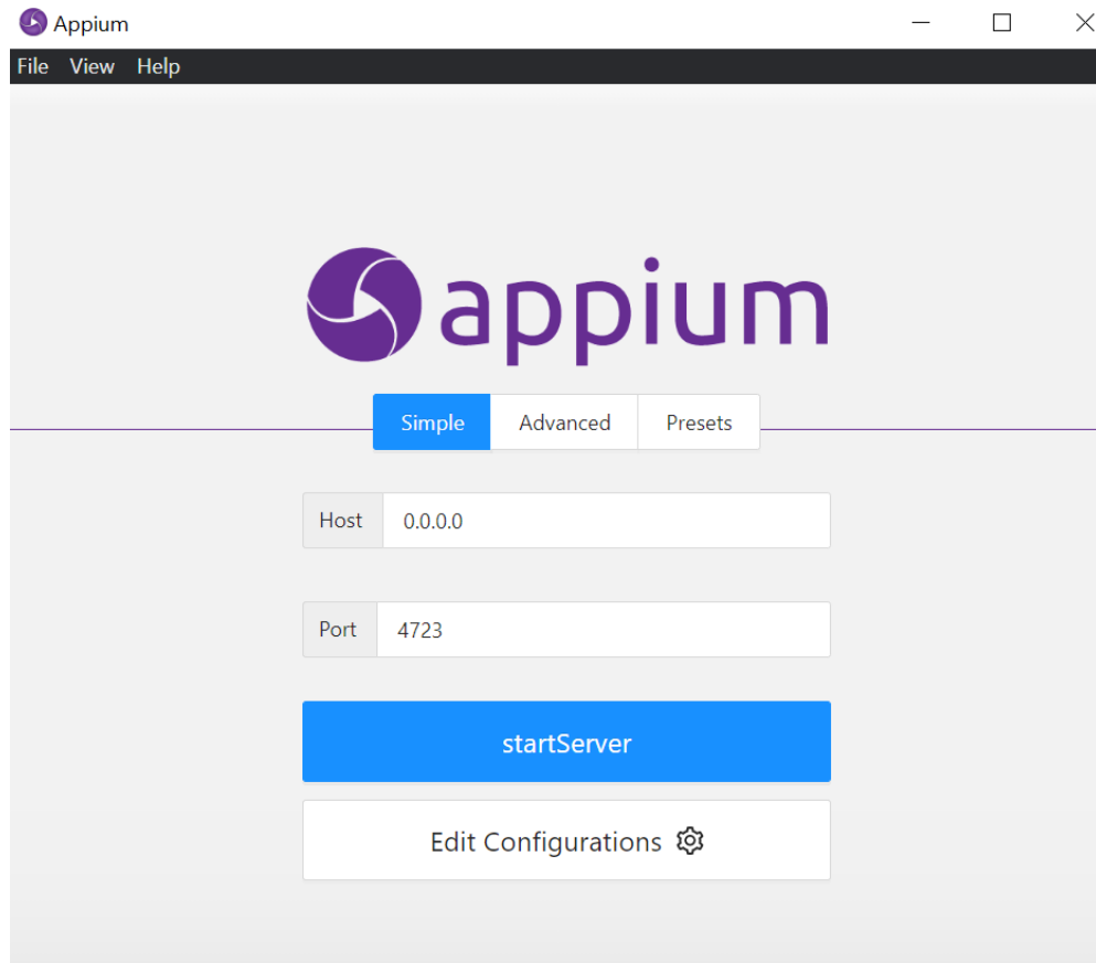
Fig 48: appium
