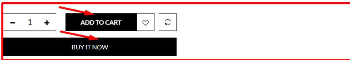
Fig 28: PD TC009
