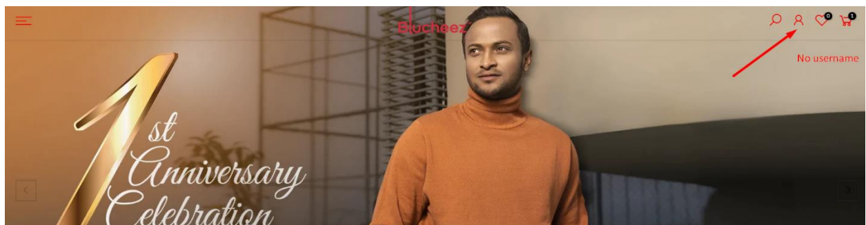
Fig 38: HP TC002
