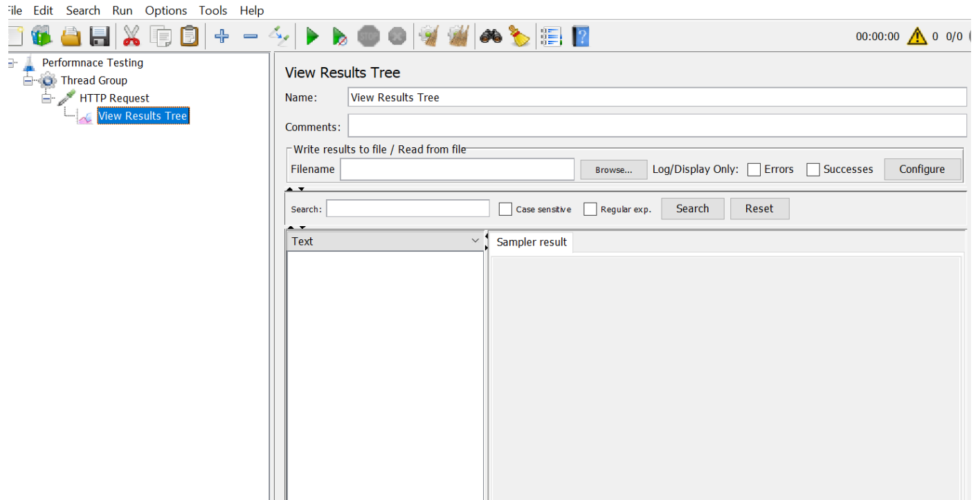
Fig 58: Run test
