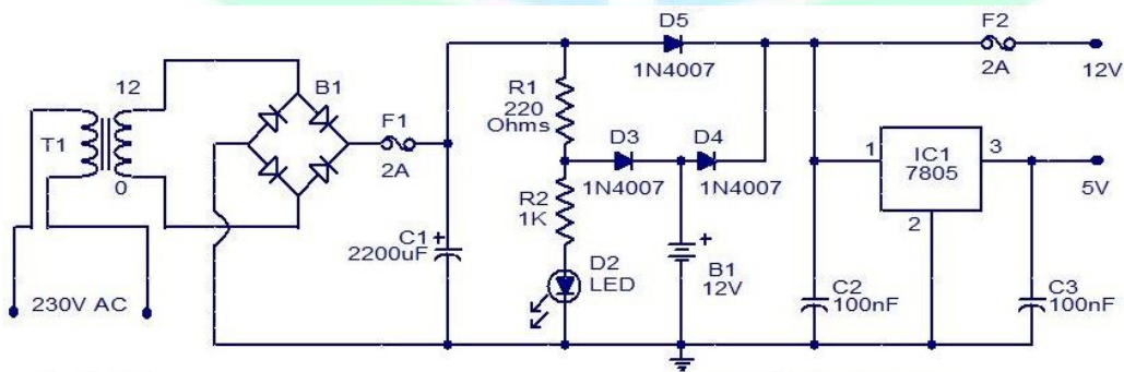
Fig 1.1 (AC to DC mini ips)
